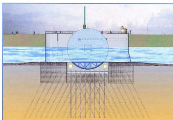
Querschnitt Hauptschiffsöffnungs
